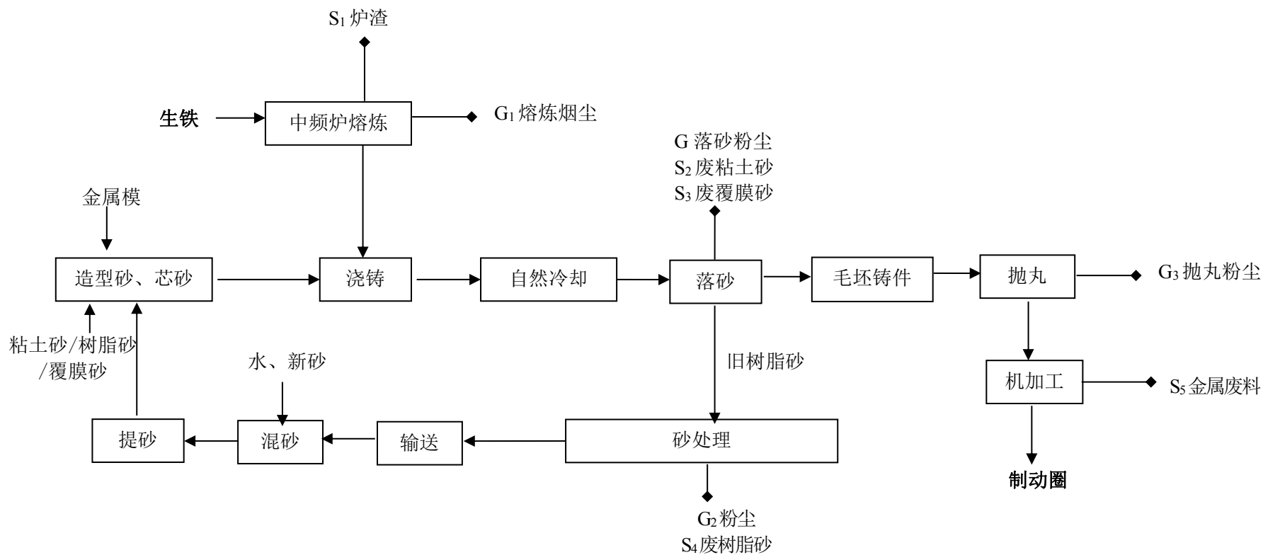
图 6-1 制动圈生产工艺流程及主要产污环节图
