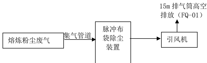
图 7-1 熔炼粉尘废气收集处理工艺流程图
