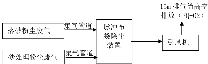
图 7-2 落砂、砂处理粉尘废气收集处理工艺流程图
