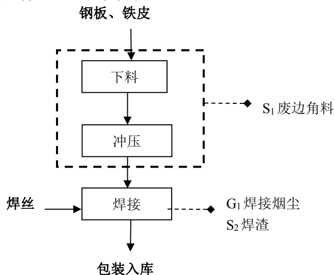
图 1 汽车钣金件生产工艺及产污环节
